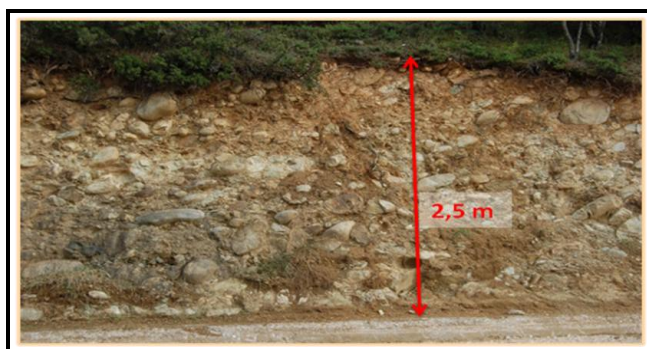
5. ábra: Útmenti feltárás: üledékes konglomerátum anyaga tanulmányozható a kolostorok felé vezető út mentén. (fotó: Dobos A.)
