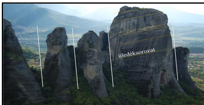
8. ábra: A különálló sziklatornyok üledéksorozatai és törésvonalai. (fotó: Dobos A.)
