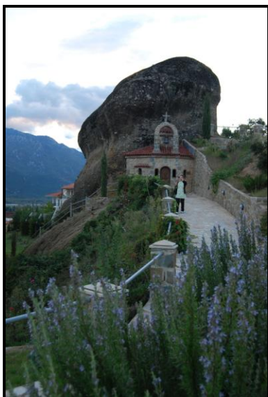
15. ábra: Kisebb kápolna és belsejére a Meteorák peremén Kalambakában. (fotó: Dobos A.)
