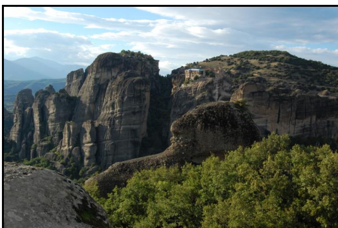
11. ábra: Csoportos sziklatornyok keletkezése. (fotó: Dobos A.)
