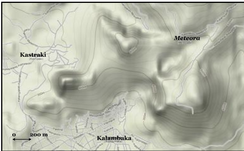
1. ábra: A Kalambakától északra fekvő Andikhasiai-hegység és a Meteorák. (Google Earth, 2010. alapján)
