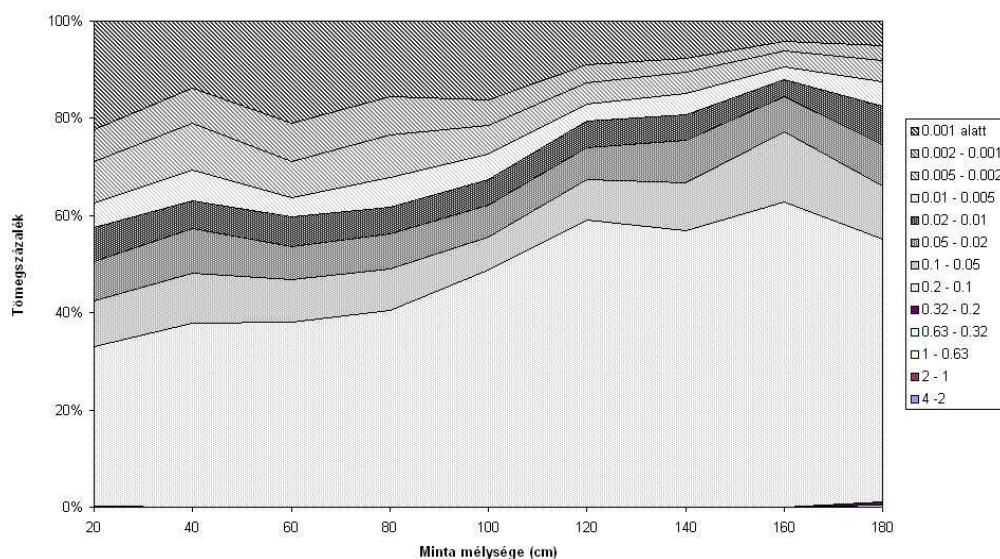
5. ábra: Cered, Mise-hegy alatti völgyváll fúrásmintájának szemcseösszetételi görbéje figure 5.: Granular composition of the borehole in the Mise Mountain (Cered)
