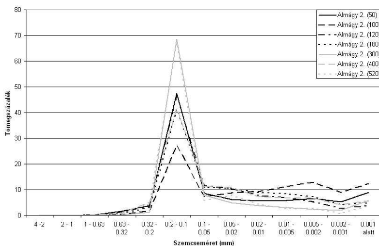
6. ábra: A dobfeneki homokbánya szemcseösszetételi görbéje figure 6.: Granular composition of the Sandmine in Dubno
