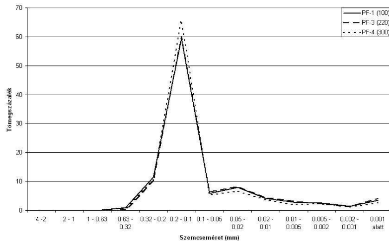
7. ábra: A Gömörpéterfala – Dobfenek - Utaspuszta útélágazás feltárásfalának szemcseösszetételi görbéje figure. 7.: Granular composition of the sample between Petrovce, Dubno and Utaspuszta
