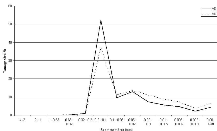
4. ábra: Az Almágy-Détér közötti földút mentén lévő útbevágások szemcseösszetételi görbéje figure. 4.: Granular composition of the samples near the road between Gemerský Jablonec and Gemerské Dechtare
