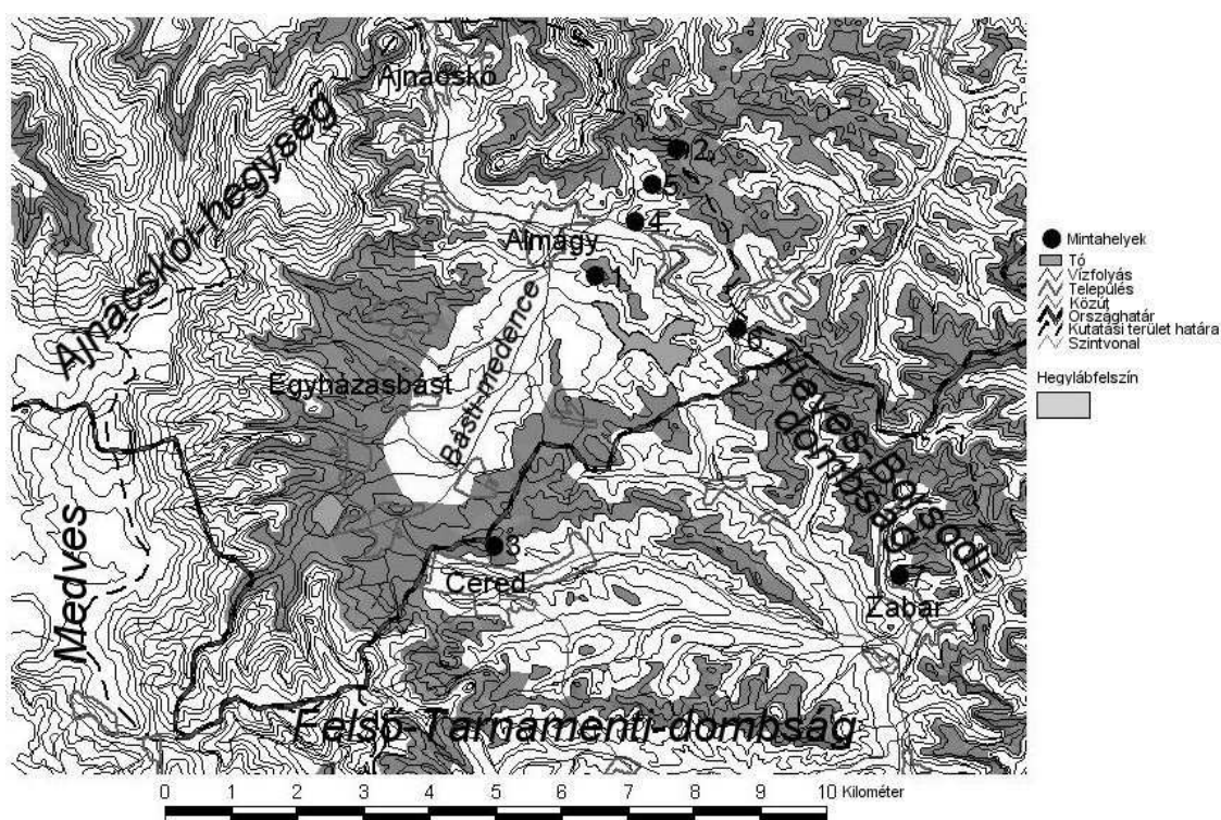
1. ábra: Hegyláb felszín a Cered-Almágyi medencében. A szürke szín a 280-330m tszf.-i magasságú övezetet (bérbaltavári hegyláb felszín) mutatja
