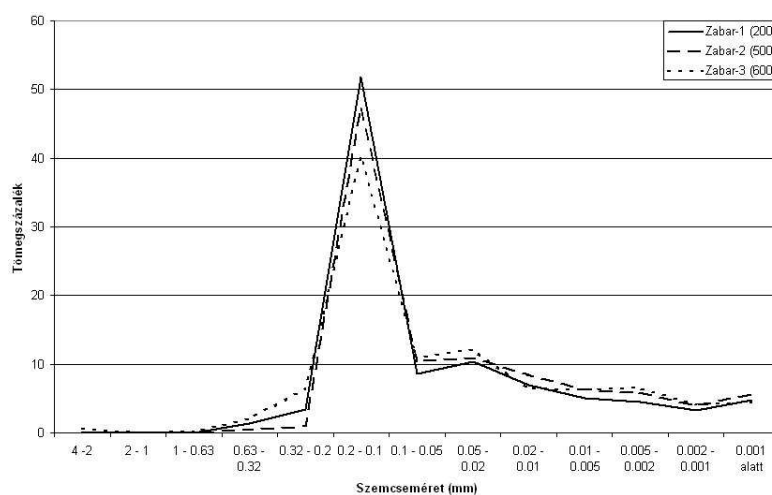
8. ábra: A Belső-Zabari-völgy feltárásfalának szemcseösszetételi görbéje figure. 8.: Granular composition of the sample in the Belső-Zabar Valley
