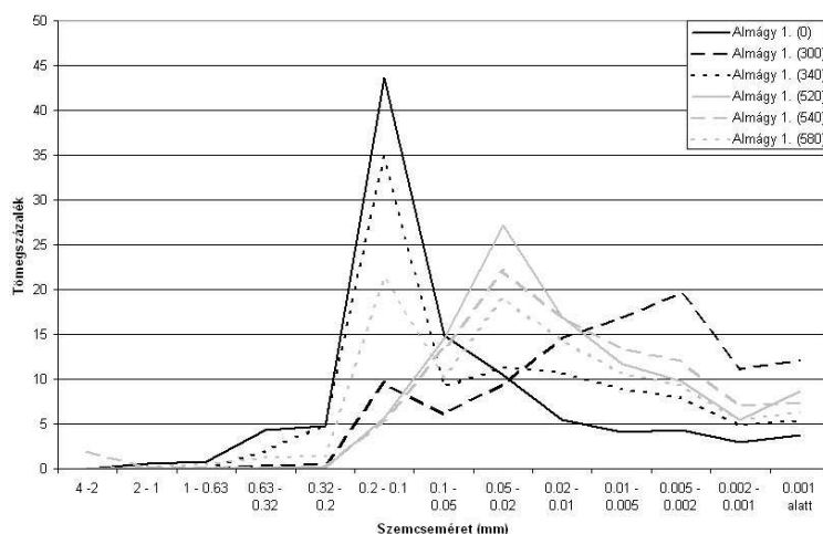
3. ábra: A csikortványhegyi bánya szemcseösszetételi görbéje figure 3.: Granular composition of the Mine in Csikortványhegy
