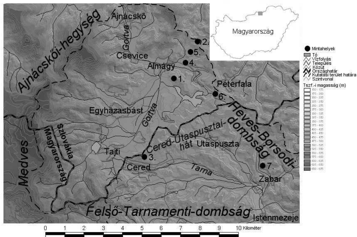
2. ábra: Mintavételi helyek a Cered-Almágyi-medencében. (A feltárások számozását lásd a szöveg alapján.) figure 2.: Samples places in the Cered-Gemerský Jablonec Basin. The numbers of the samples can be seen in the text.
